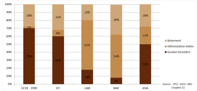
Figure 2. Potentiel technico-économique d'atténuation des types de projets forestiers par régions du monde (source GIEC - AR5)
